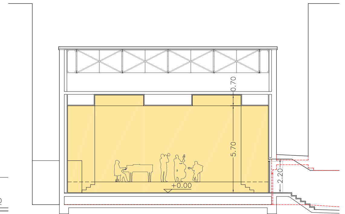
SECCIÓ TRANSVERSAL
